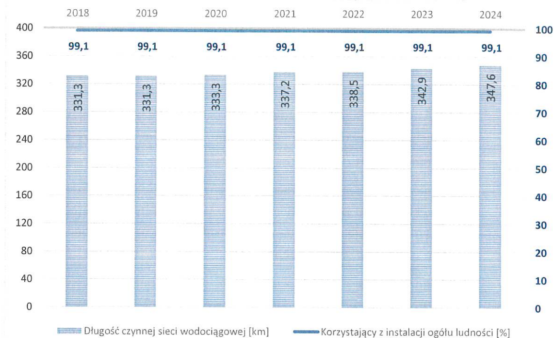
Wykres 4. Przylączy do sieci wodociągowej oraz wskaźnik zwodociągowania gminy Mogilno w latach 2018 – 2024
