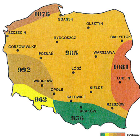
Rysunek 6 Uśłonecznienie w Polsce w kWh/m 2
