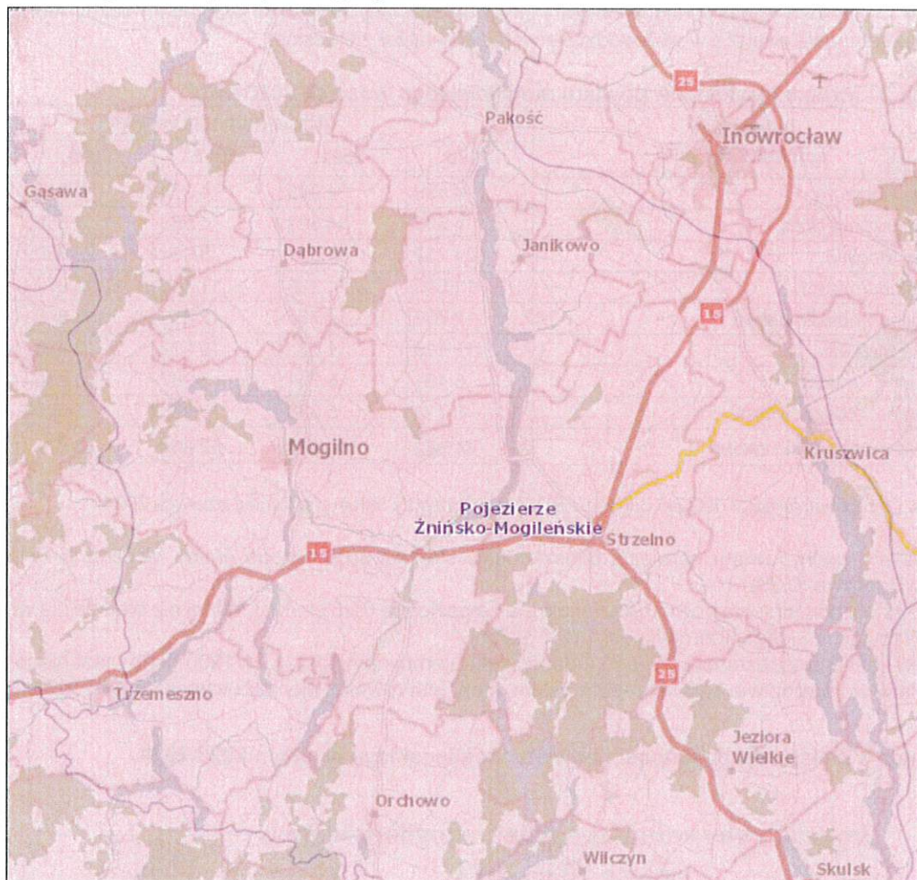
Rysunek 2 Regionalizacja fizyczno-geograficzna
