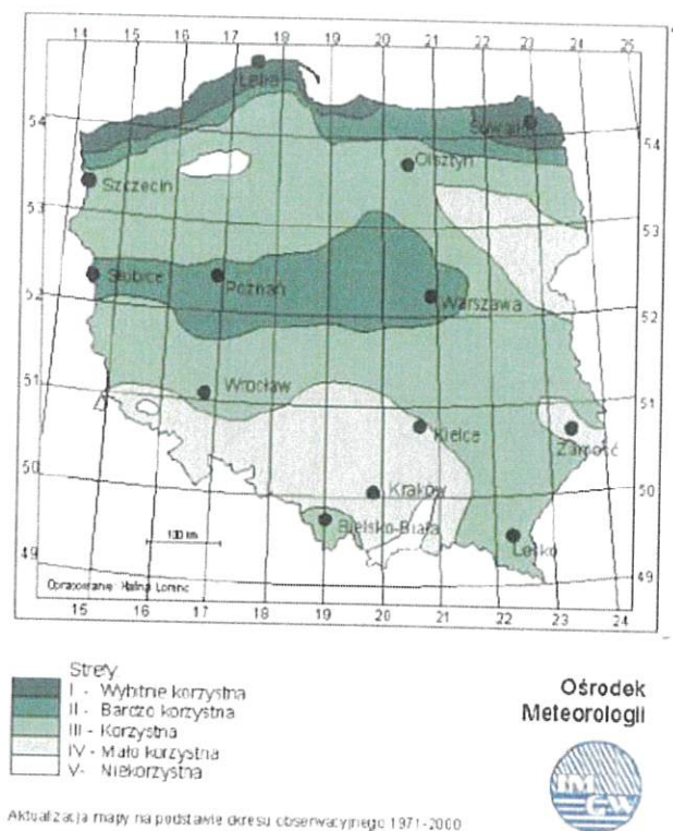
Rysunek 5 Zasoby energii wiatrowej w Polsce
